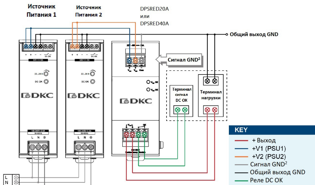
Схема подключения к резервному режиму работы
