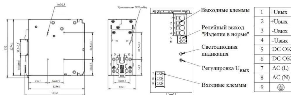
Габаритные размеры изделия
