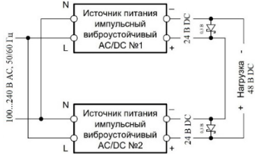
Последовательное подключение двух источников питания (с применением диодов Шоттки)
