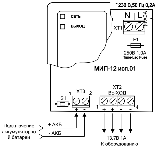
Рис. 3 Схема подключения МИП-12 исп.01 (МИП-12-1/7ПЗ)
