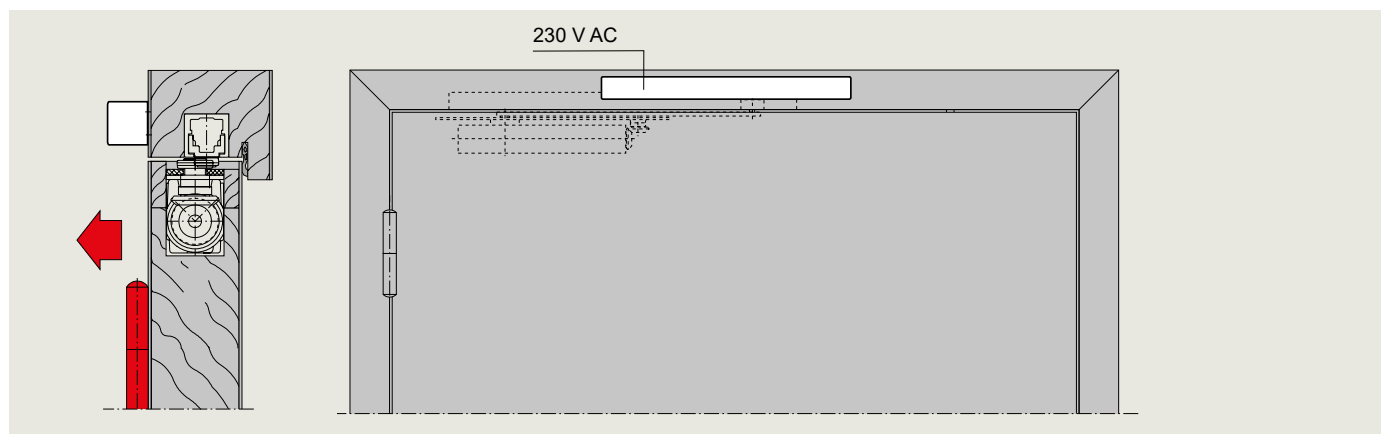
Датчики дыма пожарной сигнализации RMZ со стороны петель вместе с ITS 96 EMF Пример: дверь DIN-L, дверь DIN-R в зеркальном отражении.
