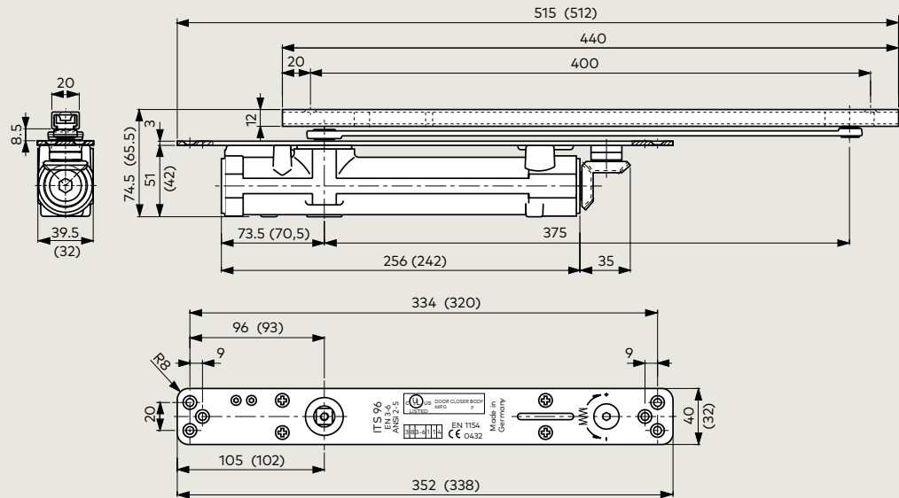
Изображение ITS 96 EN 3 – 6 ( ) размеры = ITS 96 EN 2 – 4
