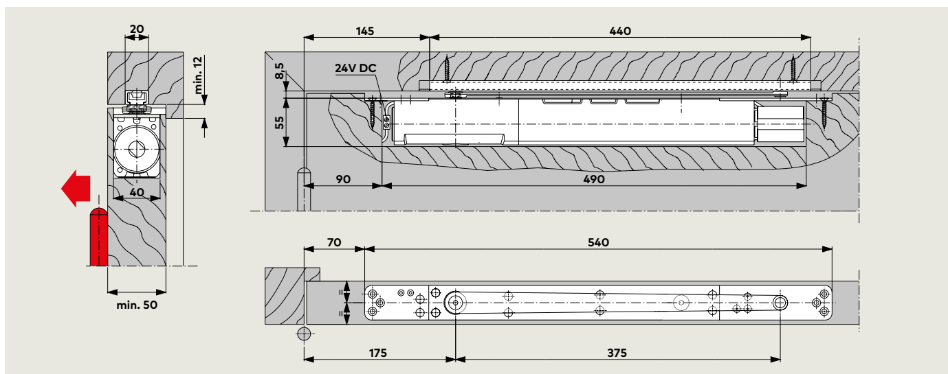
Доводчик ITS 96 FL со скользящим каналом G 96 N20 в деревянной двери
