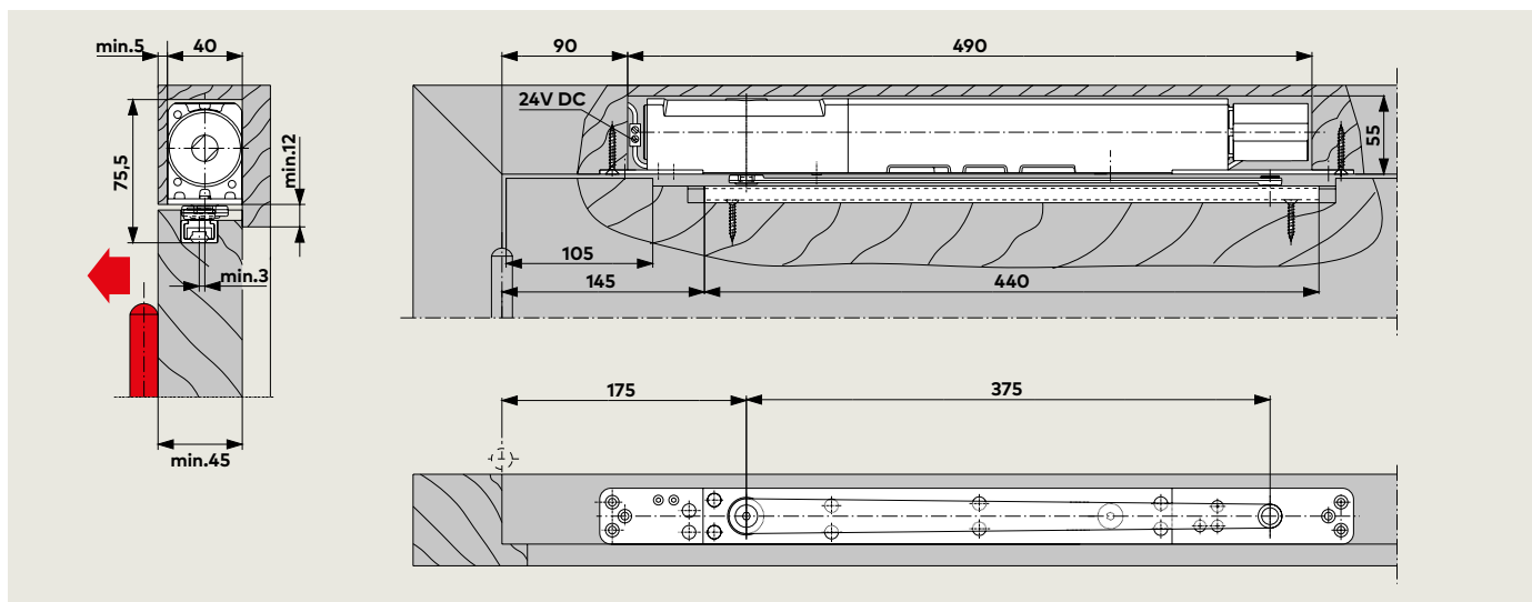
Доводчик ITS 96 FL со скользящим каналом G 96 N20 в деревянной двери с монтажом тела доводчика в коробке
