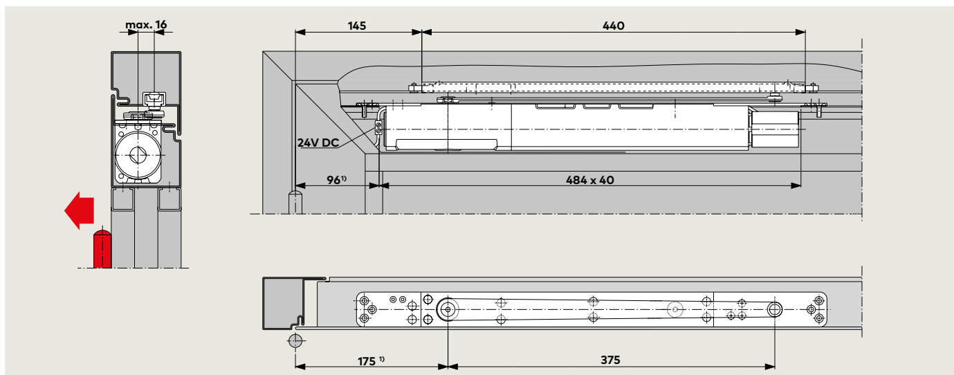
Доводчик ITS 96 FL со скользящим каналом G 96 N20 в профильной двери
