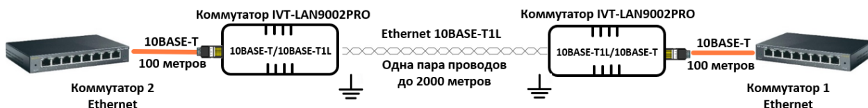
Рис. 4 Типовая схема соединения двух разнесенных сегментов сети Ethernet с помощью IVT-LAN9002PRO
