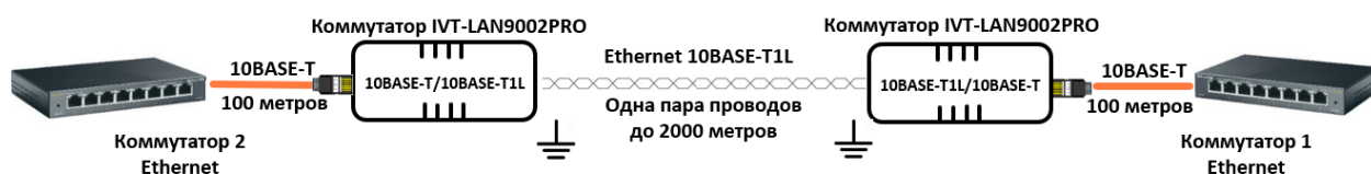
Рис. 1 Типовая схема соединения двух разнесенных сегментов сети Ethernet с помощью IVT-LAN9002PRO
