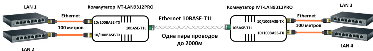
Рис. 4 Типовая схема объединения сегментов сети Ethernet с помощью Удличителя IVT-Long-IP Double по двум проводам на удаленности до 2 км. друг от друга
