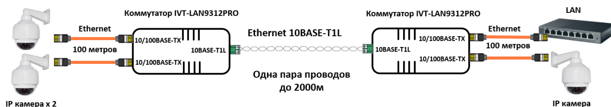
Рис. 6 Типовая схема подключения удаленных IP-камер по двум проводам (коаксиальный кабель, витая пара, другие) при модернизации
