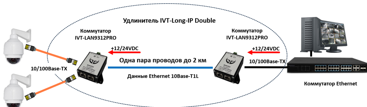
Рис 1. Схема работы Удлинителя IVT-Long-IP Double
