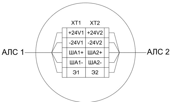
Рисунок 2 – Схема внешних подключений четырехпроводной АЛС
