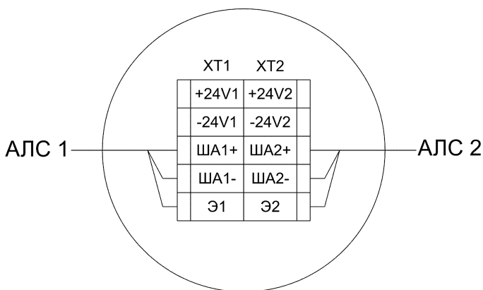
Рисунок 3 – Схема внешних подключений двухпроводной АЛС
