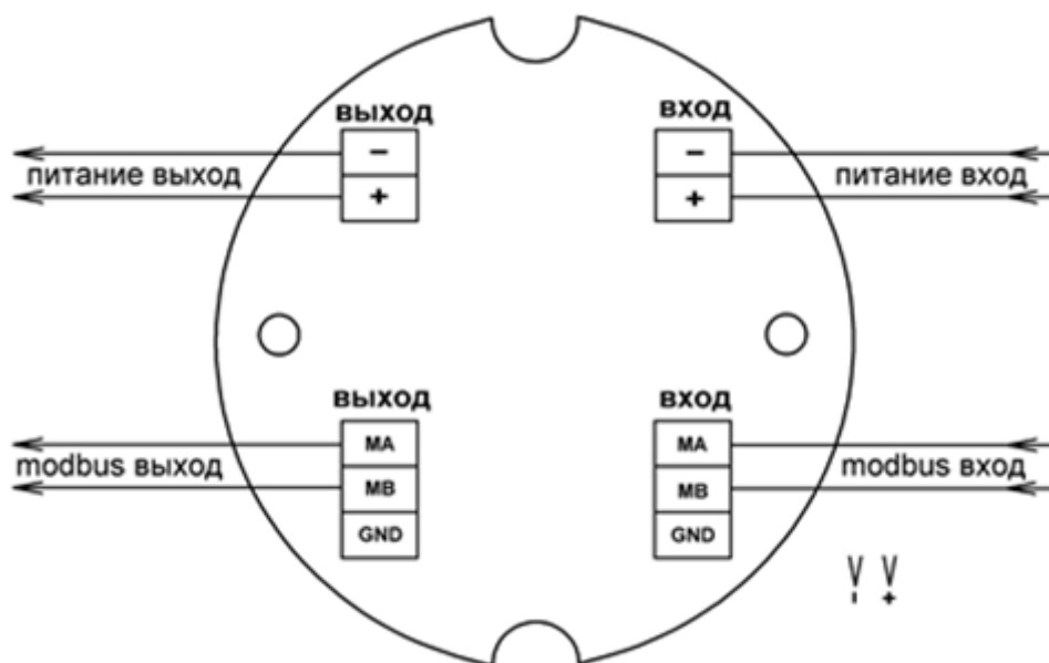
Рис. 3 – Типовая схема включения ИКЗ
