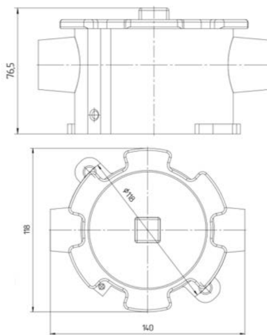
Рисунок 2 – Габаритные размеры Спектрон-ИКЗ-Modbus-Exd-H
