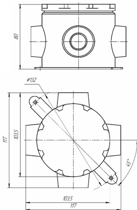
Рисунок 1 – Габаритные размеры Спектрон-ИКЗ-Modbus-Exd-A
