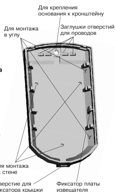
Рисунок 2 – Основание извещателя и кронштейн
