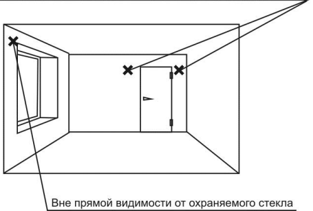
Рис.3 Запрещенные места установки
