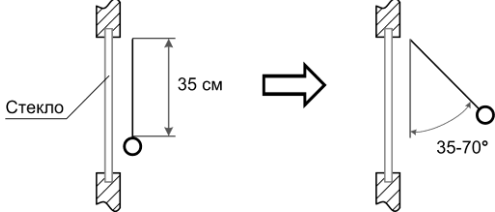
Рис.6 Тестирование извещателя
