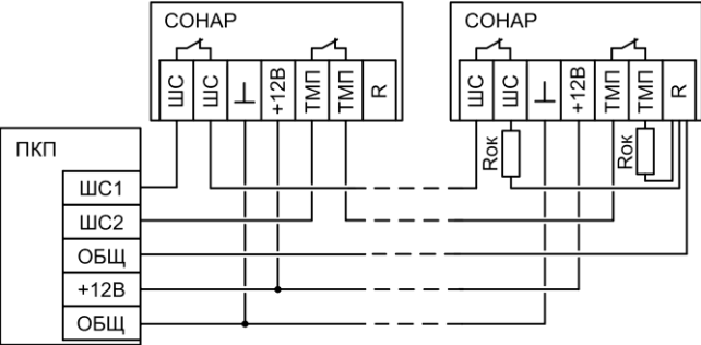
Рис.4 Схема подключения к ПКП
