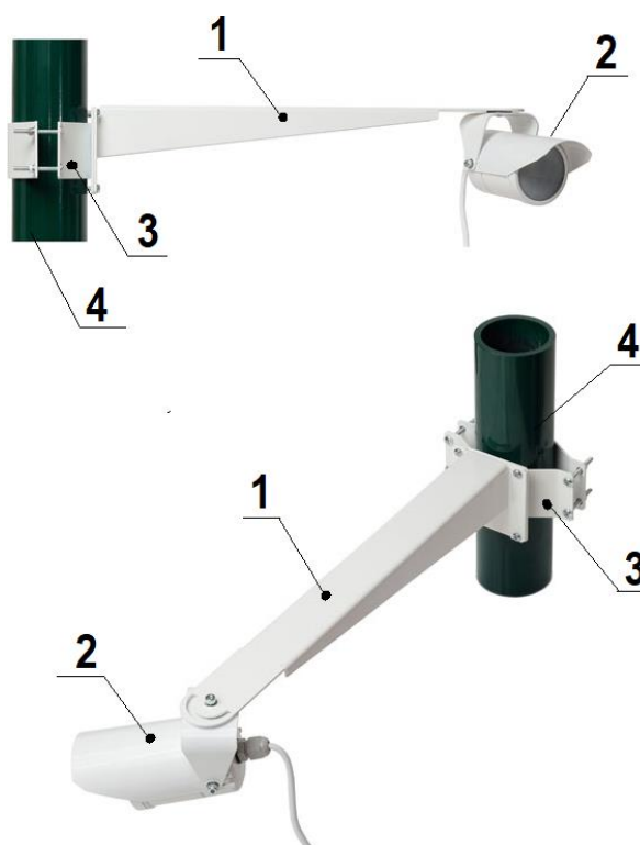
1 - кронштейн KB-949; 2 - извещатель, фиксируемый на кронштейне; 3 - кронштейн типа КТ для крепления к трубе; 4 - труба
