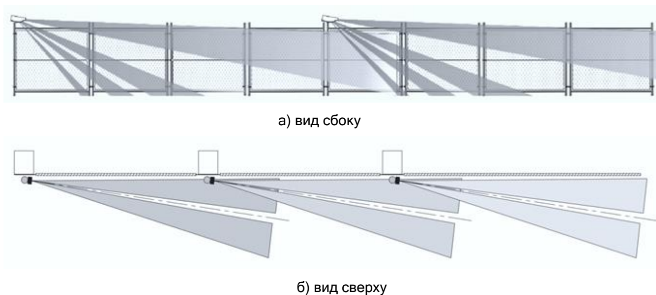
Рисунок 2.1 - Однонаправленная схема установки извещателей
