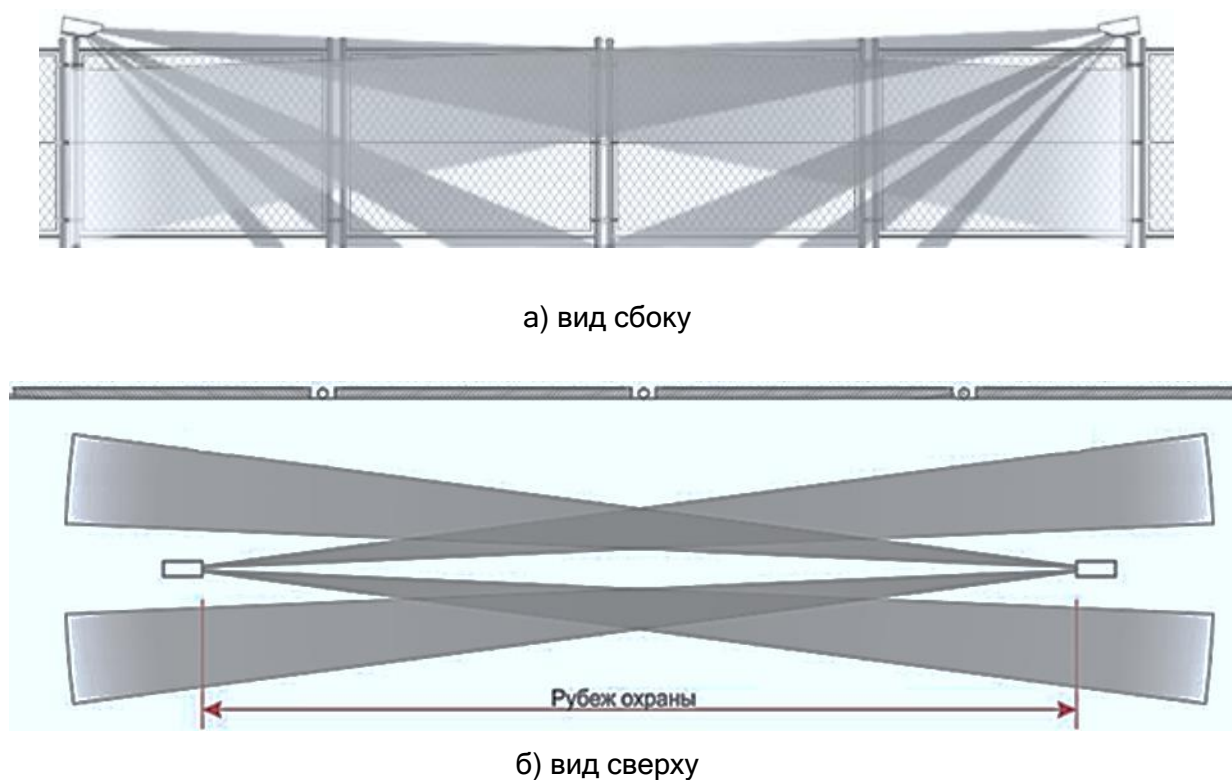
Рисунок 2.2 - Двухнаправленная схема установки извещателей
