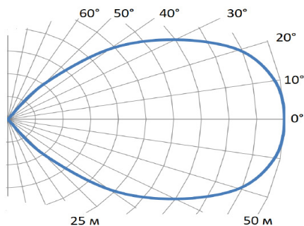
Рисунок 58 – Диаграмма обнаружения в любой плоскости
