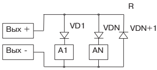
Рисунок 29 – Схема подключения исполнительных устройств к БКВ-Ех
