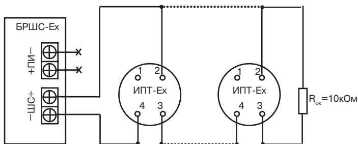
Рисунок 55 — Рекомендуемая схема подключения ИПТ-Ех к БРШС-Ех (в один шлейф БРШС-Ех рекомендуеся включать не более 10 ИПТ-Ех)
