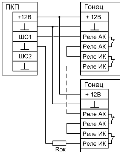
Рис.6б Схема подключения извещателей к ПКП (вариант 2)
