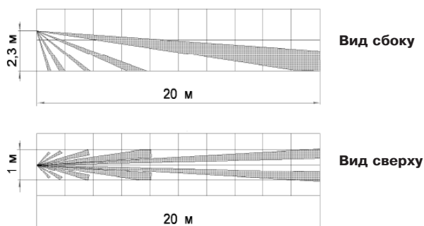
Рисунок 1 – Диаграмма зоны обнаружения
