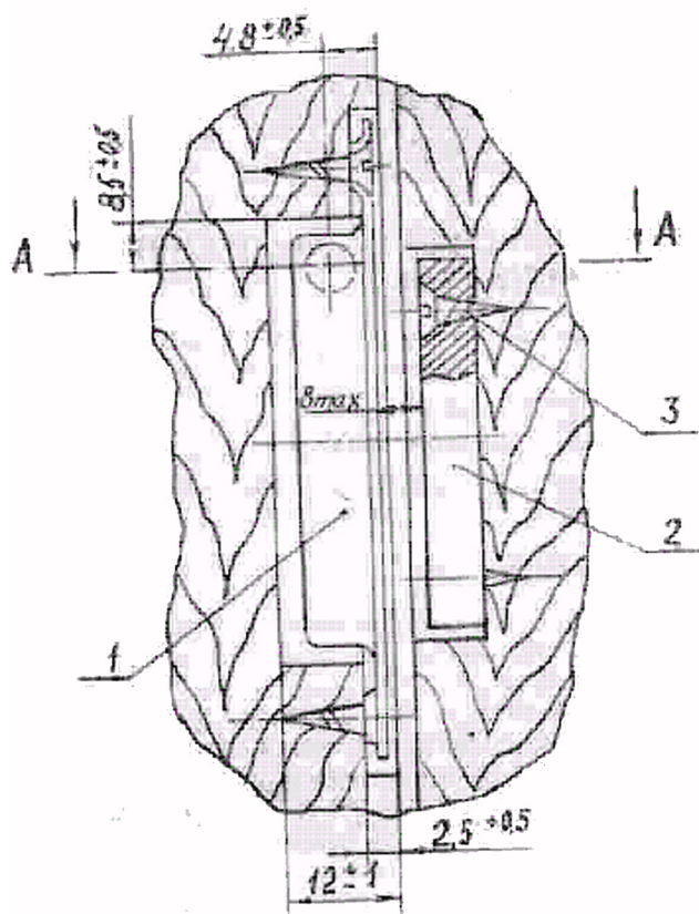
Разметка под крепление контакта поз.1
