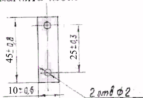
Разметка под крепление магнита поз.2
