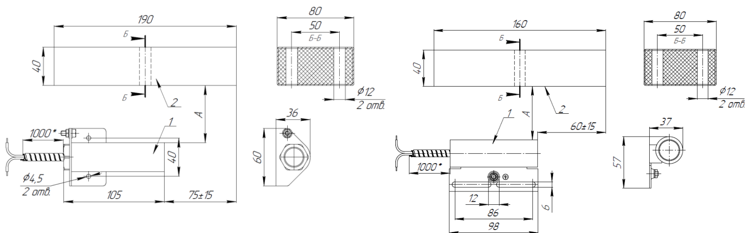
Торцевая крепежная площадка Т (съёмная)
