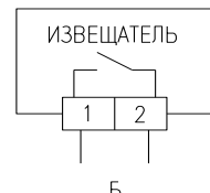
Рисунок Г. Электрическая схема датчика. Выходы датчика: 1 – красный (коричневый), 2 – черный (зеленый), 3 – синий. (прозрачный)
