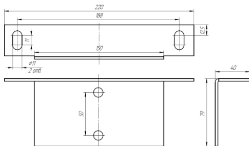
кронштейн К-02
