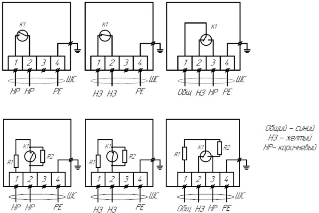
Рис.4 Конструкция и варианты кабельных вводов датчиков Ех ИО 102
