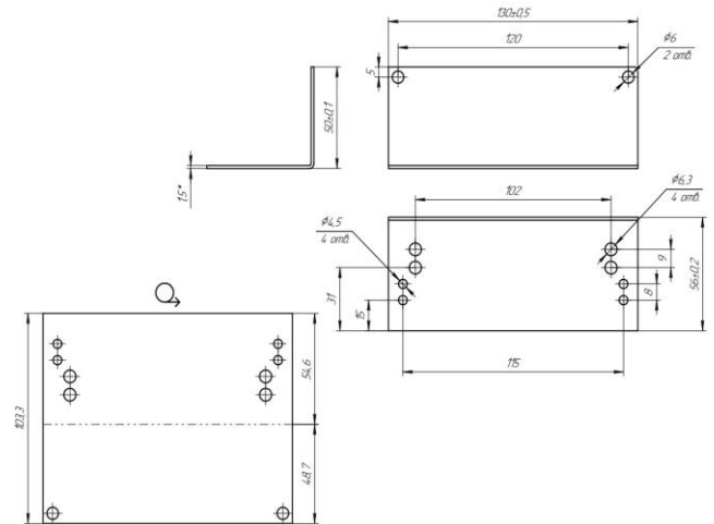
Габаритные и присоединительные размеры кронштейна К-2-100/200 АЯКС
