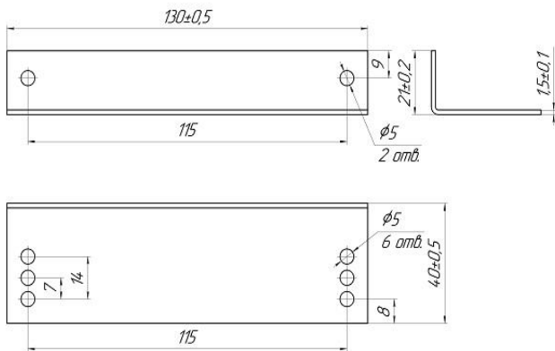
Габаритные и присоединительные размеры кронштейна К-26 АЯКС
