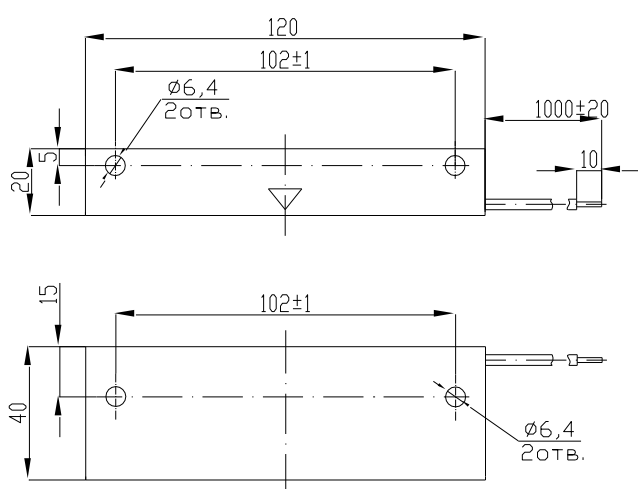
Блок геркона
