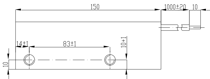
Блок геркона
