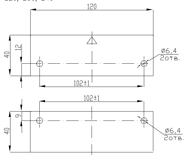
Блок магнита
