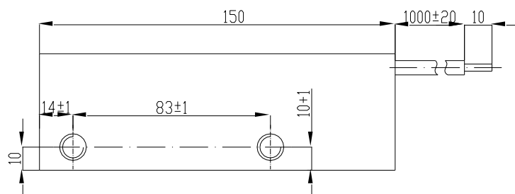
Блок геркона
