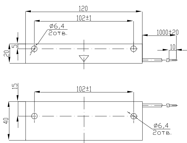
Блок геркона
