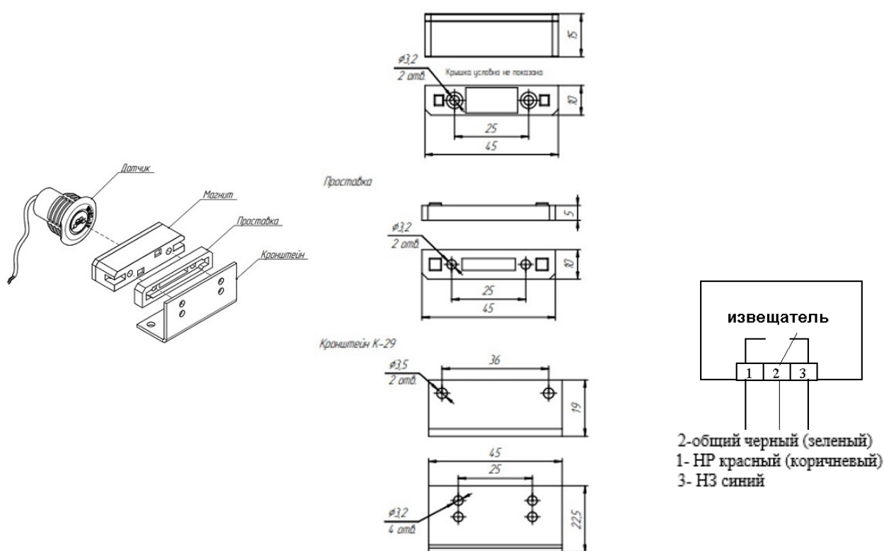
Рис.2 Габаритные размеры блока магнита в сборе с проставками и кронштейном
