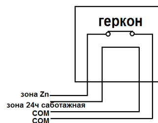
Рис.4 Схемы включения ИО102-50 «Антисаботаж»
