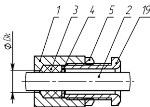
д) открытая прокладка кабеля в кабельном вводе КВБ
