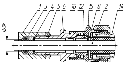
з) монтаж бронированным кабелем в металлорукаве в кабельном вводе KBВМ
