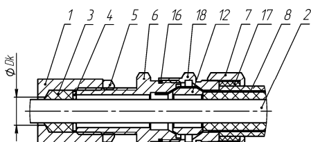
ж) монтаж бронированным кабелем в кабельном вводе KBВУ
