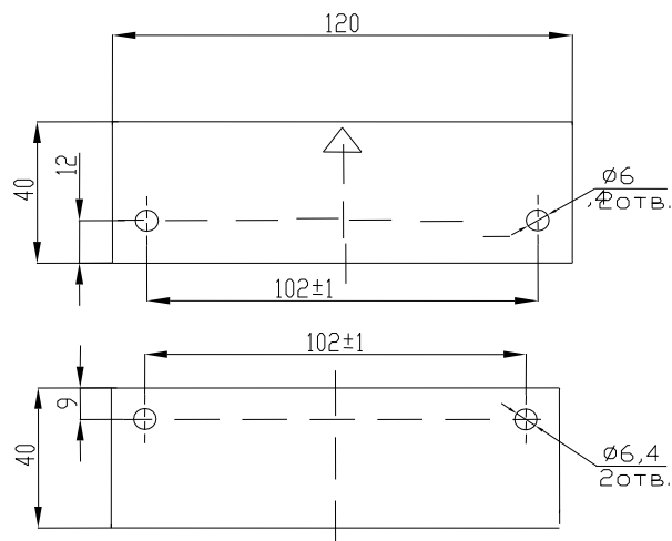
Блок магнита
