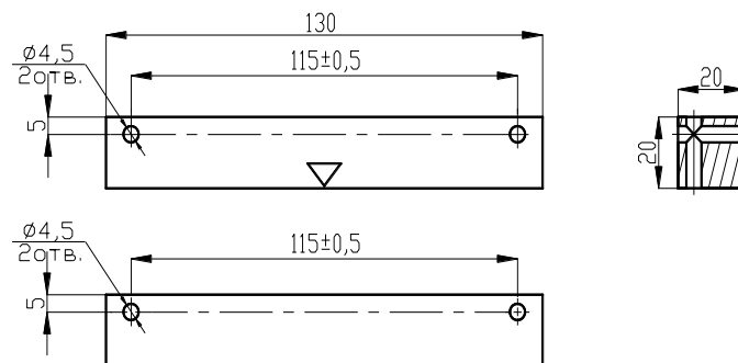
Блок магнита
