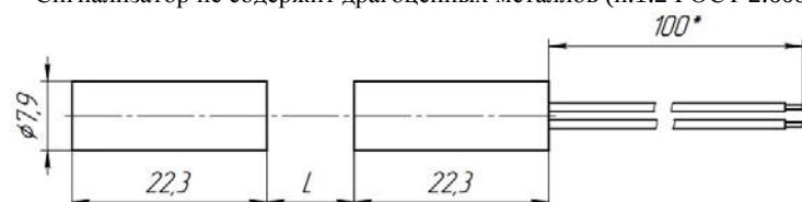
Рис.1 Габаритные размеры.
