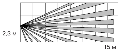
Рисунок 2 – Диаграмма зоны обнаружения извещателя «Фотон-12Б-РК»
