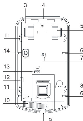
Рисунок 3 – Конструкция «Фотон-12-РК», «Фотон-12Б-РК»
