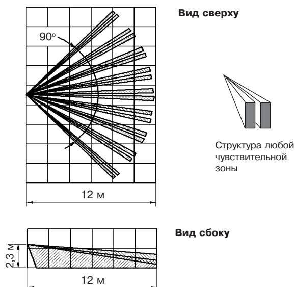
Рисунок 2 – Диаграмма зоны обнаружения
