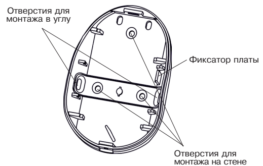
Рисунок 2 – Основание извещателя
