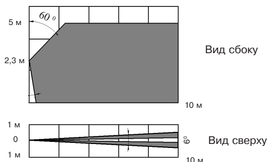
Рисунок 2 – Диаграмма зоны обнаружения извещателя «С2000-ИК» исп.04
