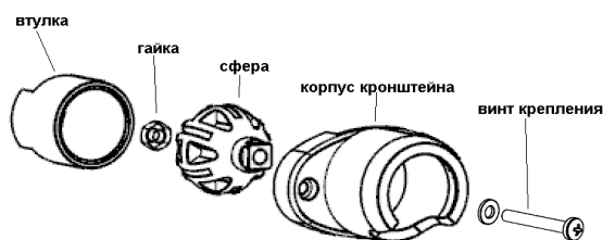
Рисунок 4 – Конструкция кронштейна
