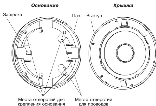
Рисунок 2 — Основание и крышка извещателя
