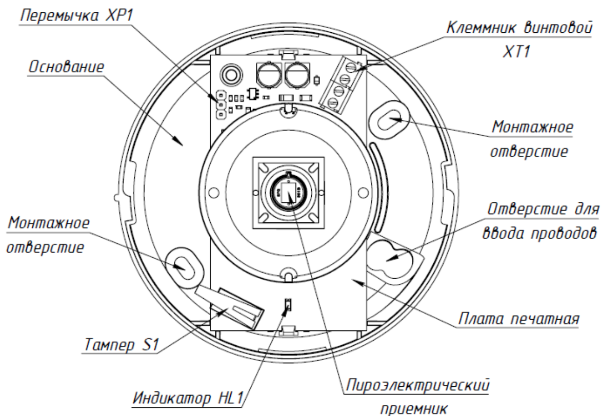
Рис.2.2.2.1. Конструкция извещателя.
