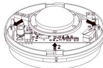
Рис.2.2.3.2.3. Схема снятия печатной платы
