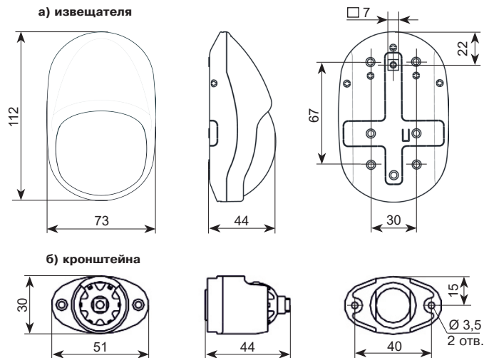
Рисунок 3 – Габаритные и установочные размеры
