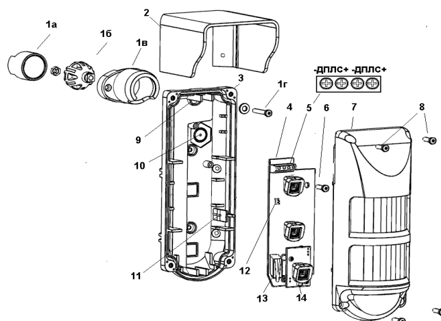
Рисунок 1 – Конструкция извещателя
