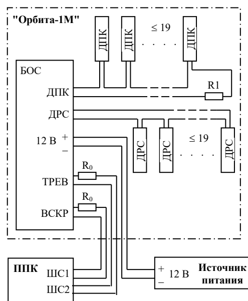
Рис. 5 – Схема подключения извещателя "Орбита-1М" с раздельной передачей извещений о тревоге и вскрытии корпуса (по двум ИШС)
