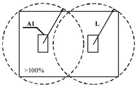
Рис.4 Полная защита конструкции
