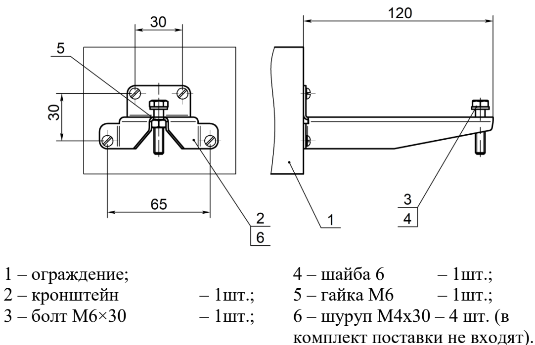
Рисунок 2.7 – Установка кронштейна 120 мм
