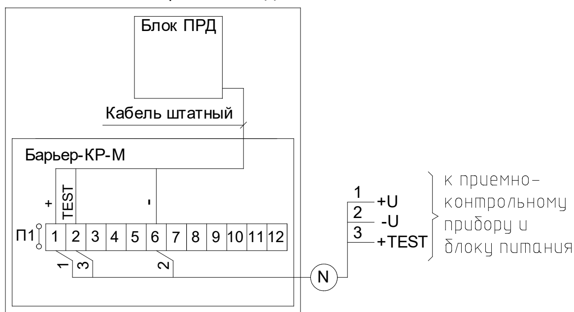
Рисунок 2.5 – Схема подключения блока ПРД при использовании распределительной коробки «БАРЬЕР-КР-М»
