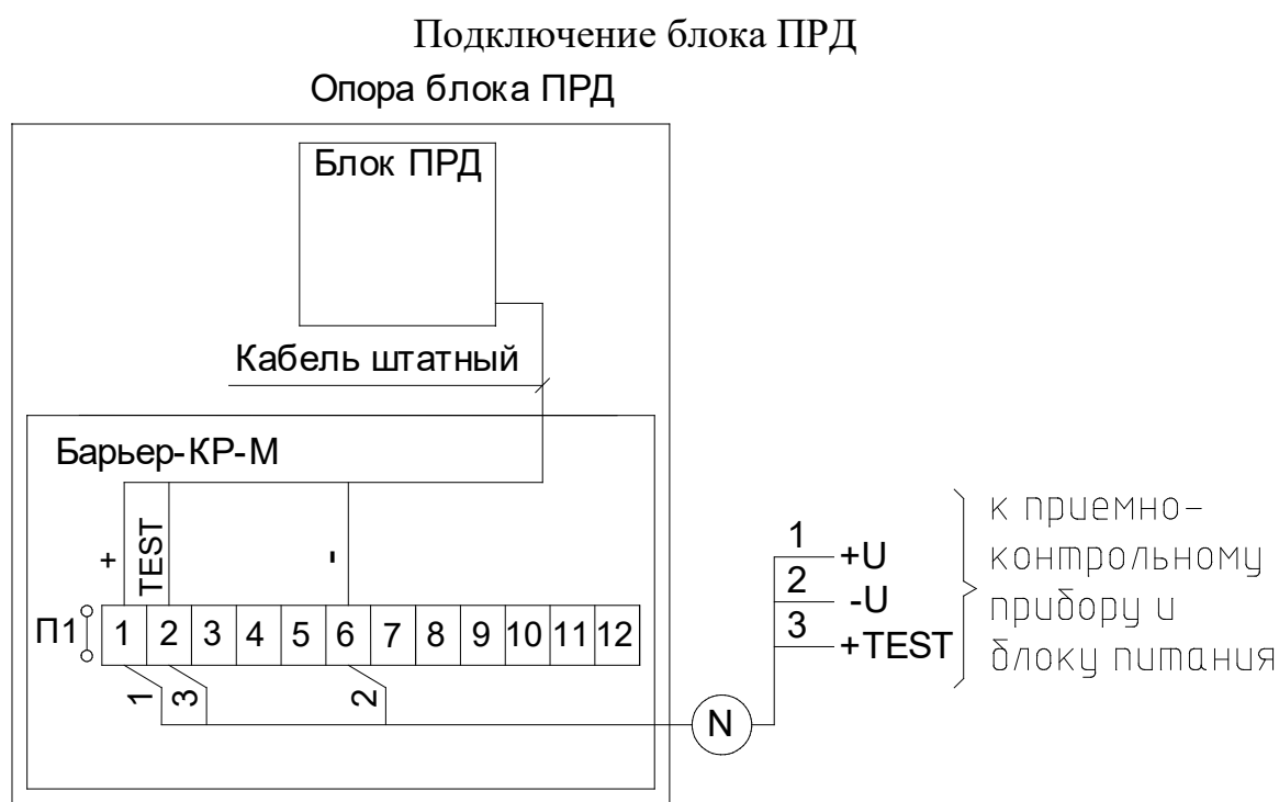
Рисунок 2.5 – Схема подключения блока ПРД при использовании распределительной коробки «БАРЬЕР-КР-М»
