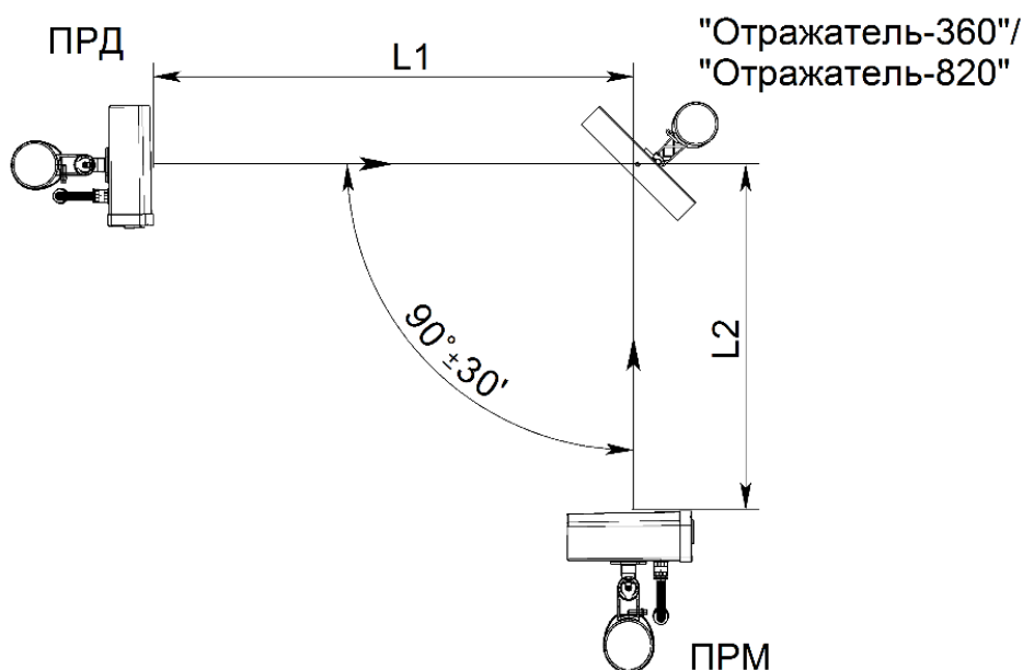
Рисунок 2.13 – Установка извещателей с применением отражателя «Отражатель-360» («Отражатель-820»)
