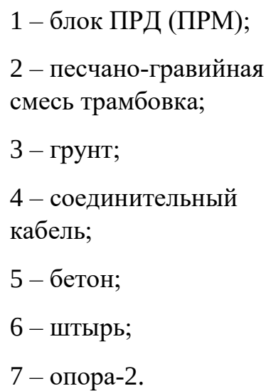
Рисунок 5.2 – Вариант установки извещателя на круглую опору в грунте.
