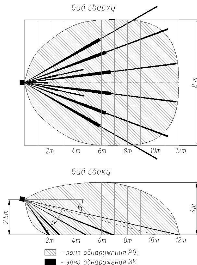
Рисунок 3.1 – Размеры зоны обнаружения извещателя «Циклоп-10»
