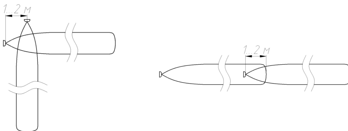
Рисунок 2.5 – Установка извещателей «с перекрытием»
