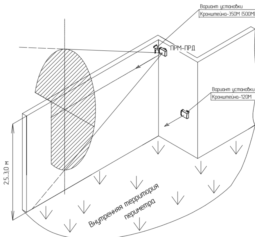
Рисунок 2.4 - Примеры установки извещателя с применением выносных кронштейнов 500, 350, 120М
