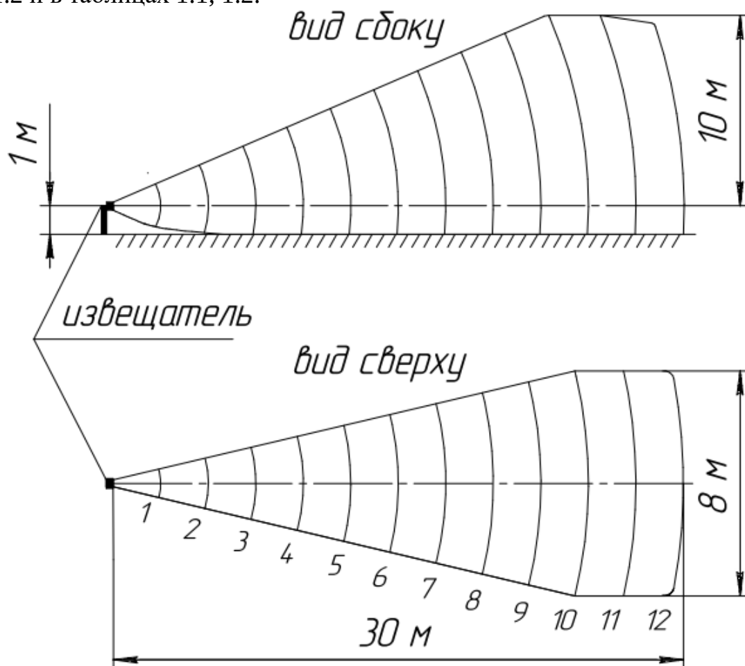
Рисунок 1.1 – Максимальная зона обнаружения, формируемая извещателями «ЗЕБРА-30(5,8)-О», «ЗЕБРА-30(5,8)-О-А», установленными на опоре, на высоте 1 метр от поверхности земли
