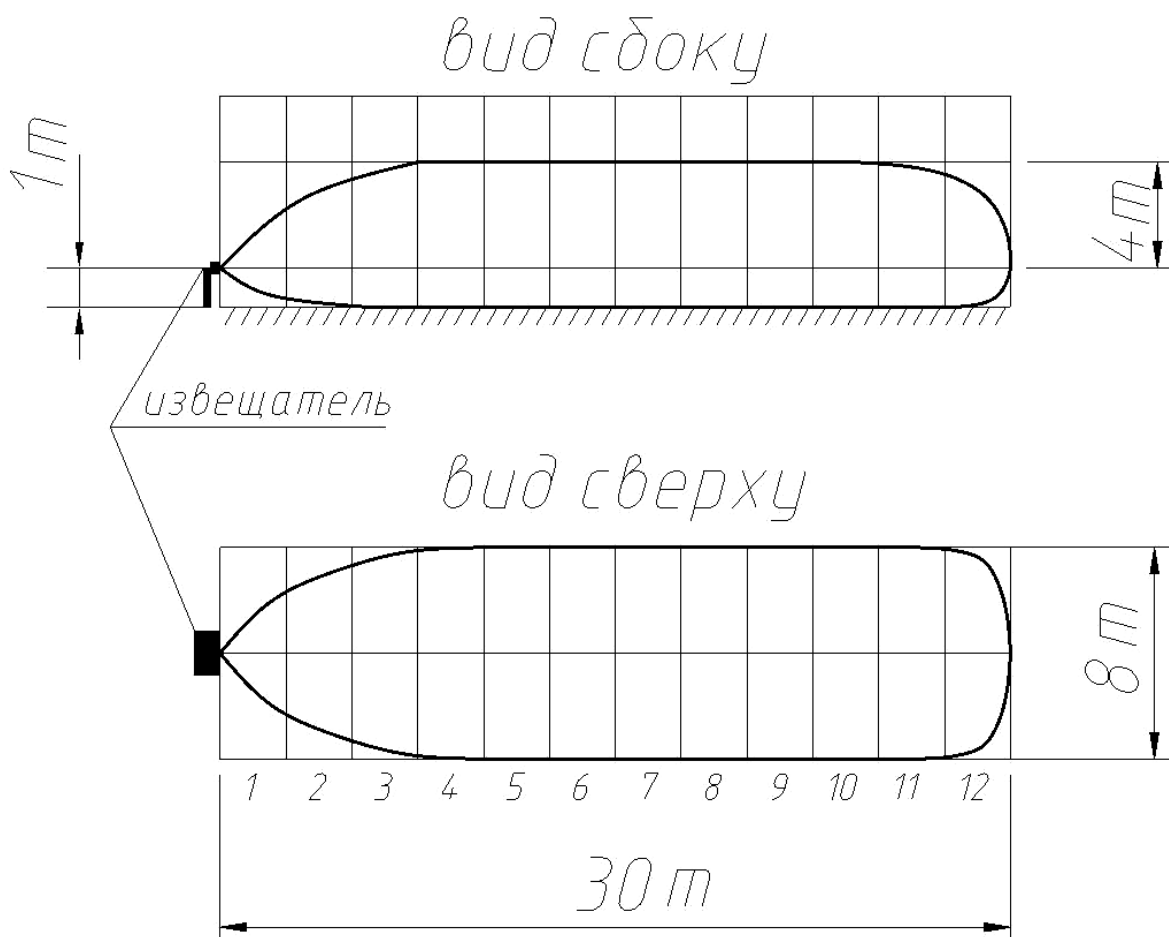
Рисунок 12.1 Зона обнаружения извещателя при установке на участке периметра на высоте 1 метр.
